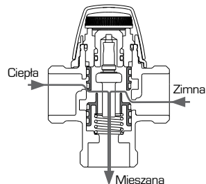
VTA350
